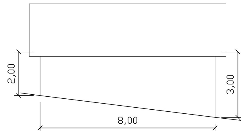
Prospetto nord
