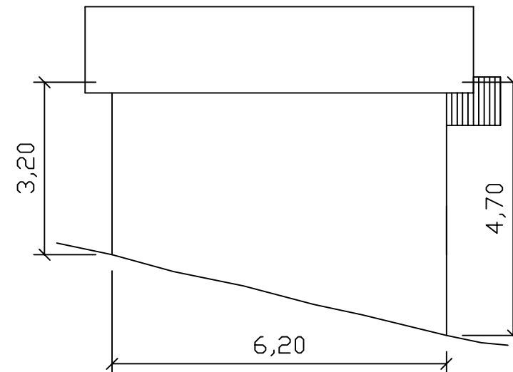
Prospetto nord
