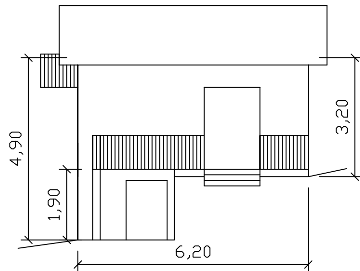
Prospetto sud
