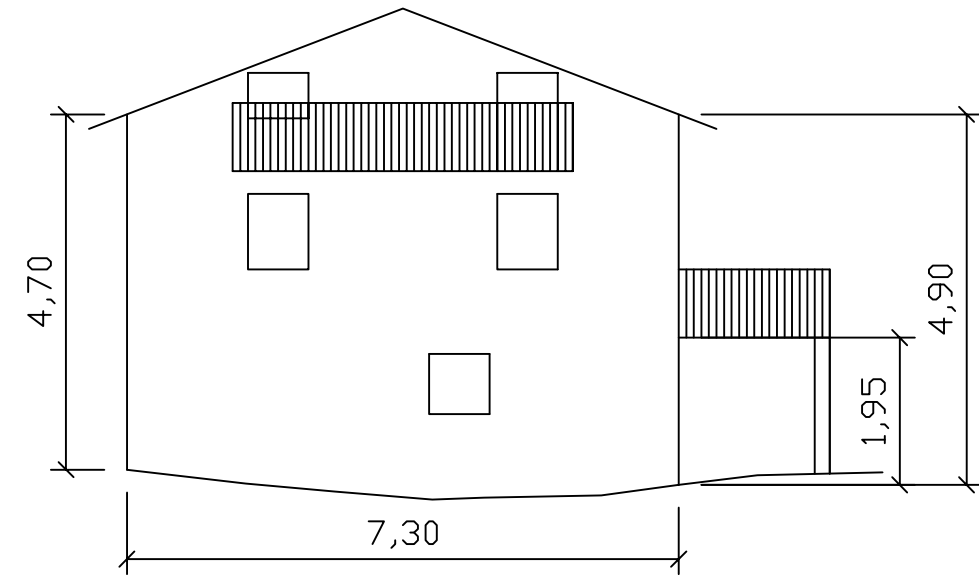
Prospetto ovest
