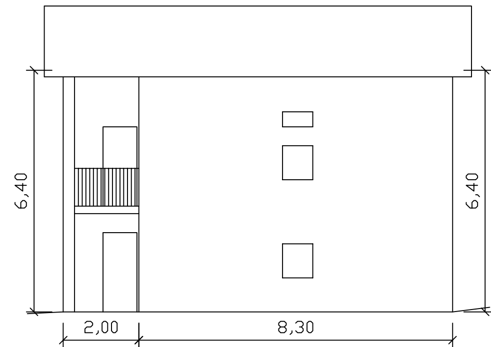
Prospetto ovest
