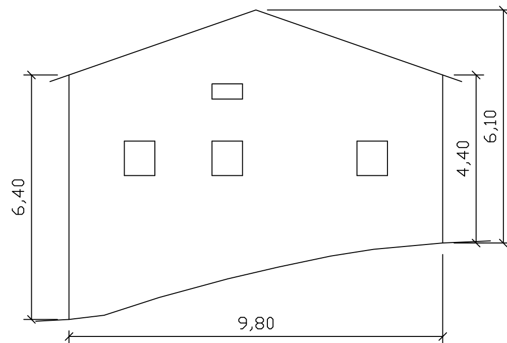
Prospetto sud
