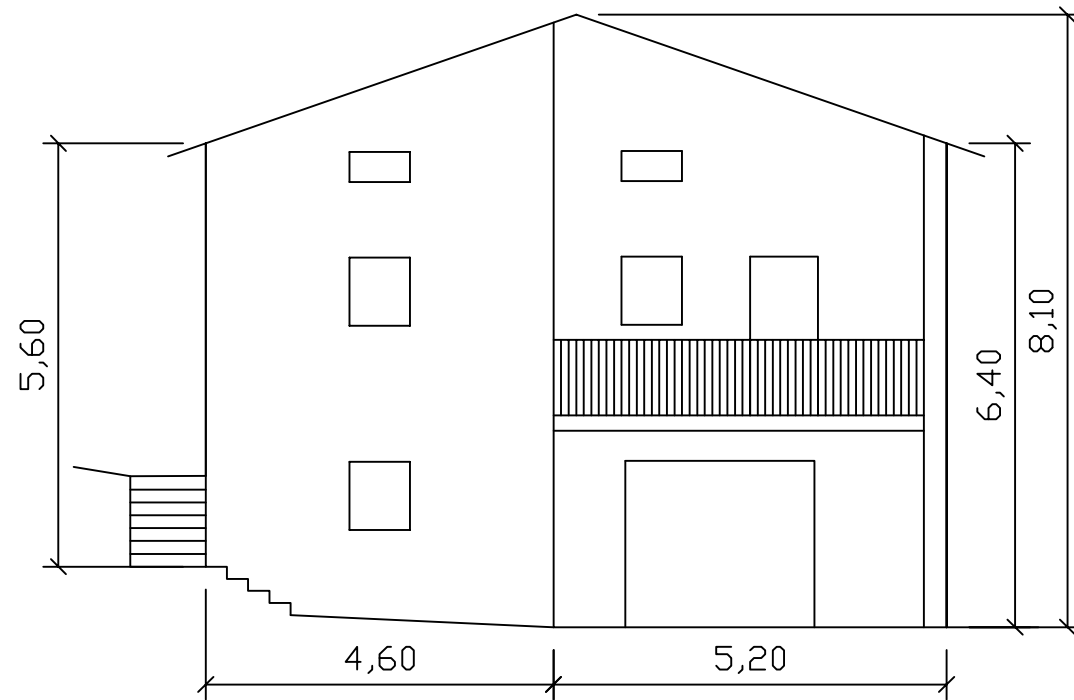
Prospetto sud
