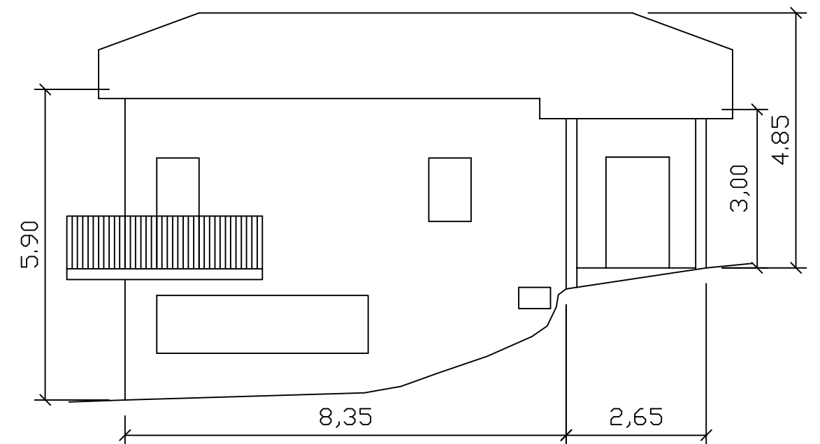
Prospetto ovest
