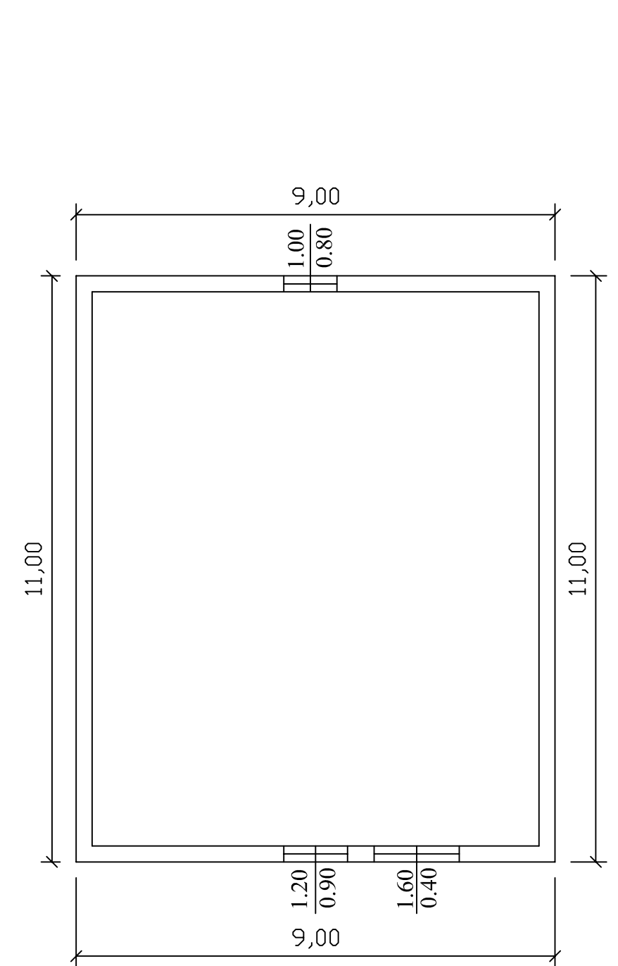
Pianta piano terzo
