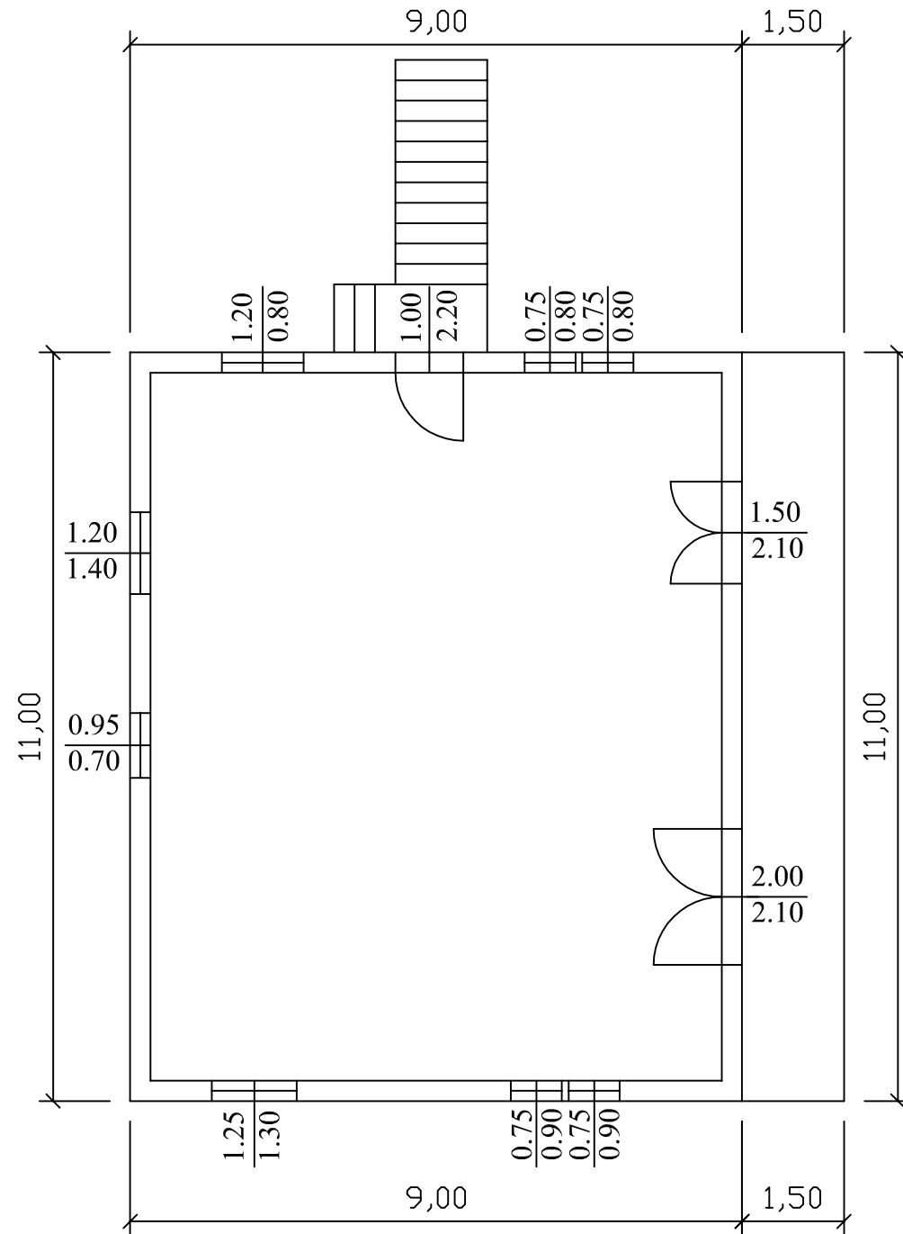
Pianta piano secondo
