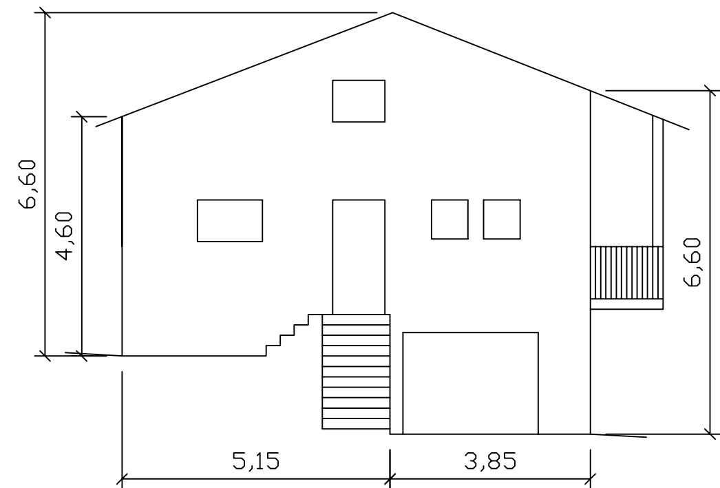
Prospetto sud
