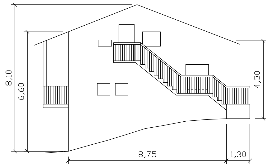
Prospetto nord
