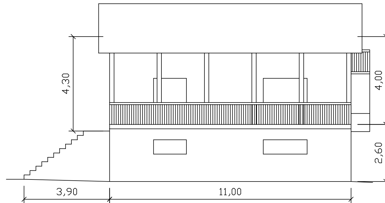
Prospetto est
