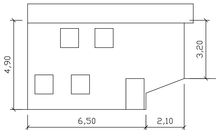
Prospetto sud
