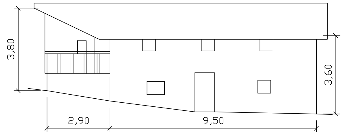
Prospetto sud
