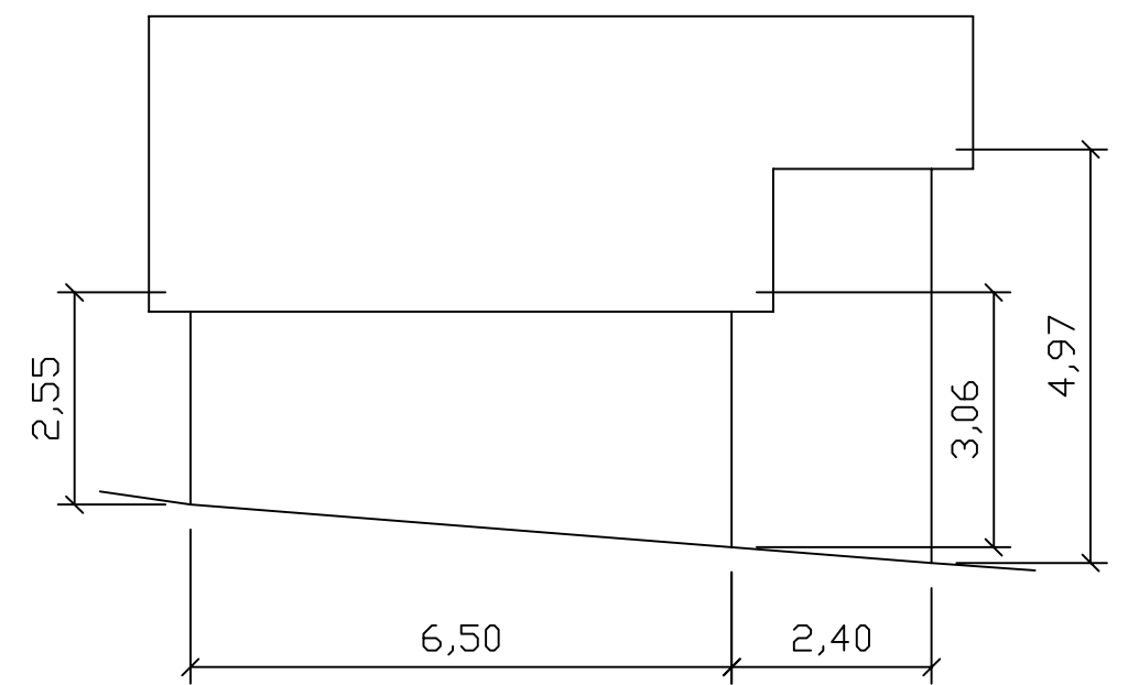
Prospetto ovest
