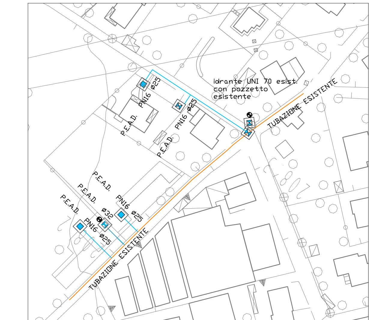
via mascagni scala 1:1000
