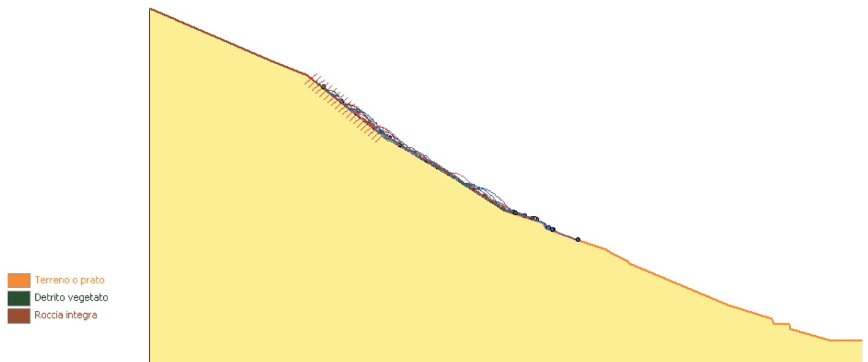
Sezione 1 - Blocco modale - 20 traiettorie
