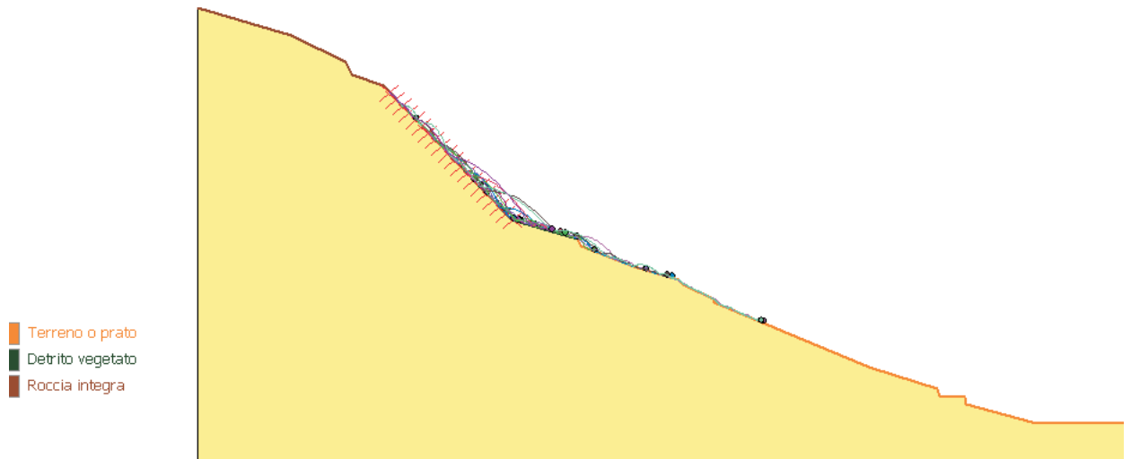
Sezione 1,5 - Blocco modale - 20 traiettorie
