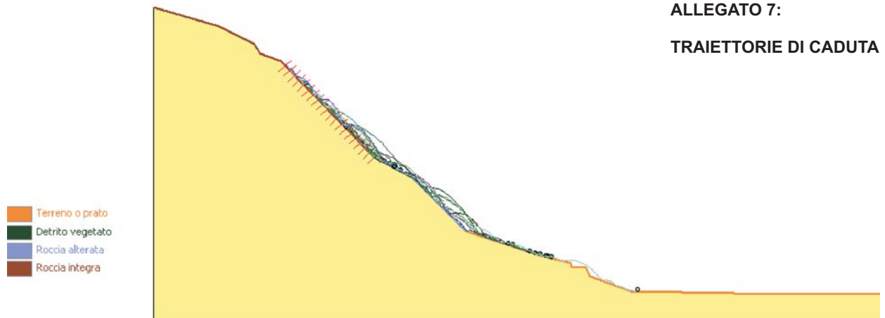
Sezione 2 - Blocco modale - 20 traiettorie
