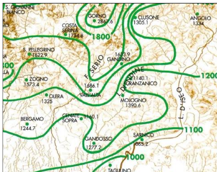
Carta delle isoiete annue (Fonte: Storia Economica e Sociale di Bergamo)
