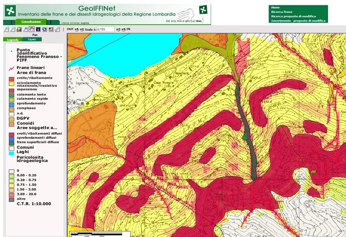
Estratto cartografia GeoIFFI con evidenziate le aree suscettibili a franosità
