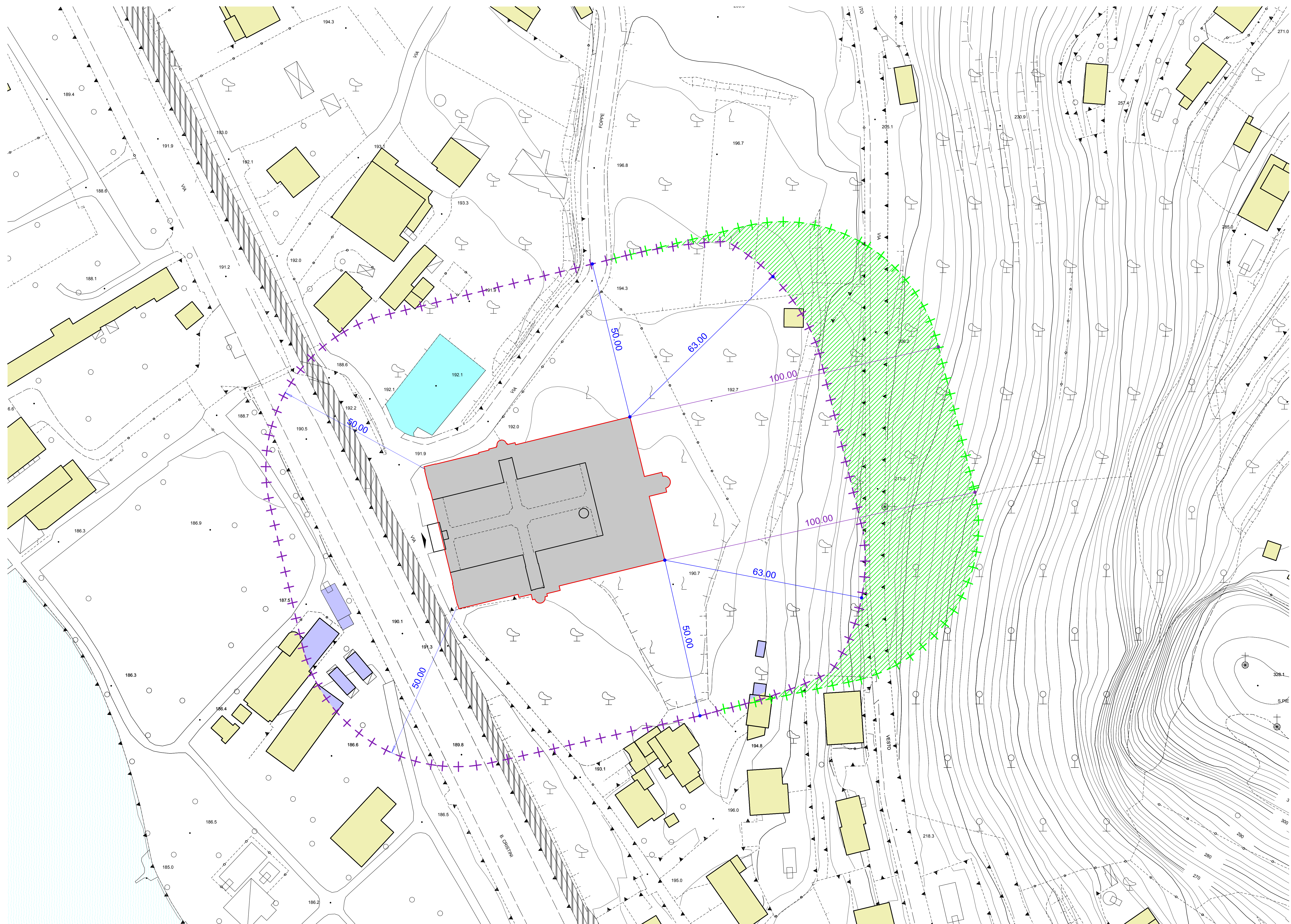
planimetria scala 1:500
