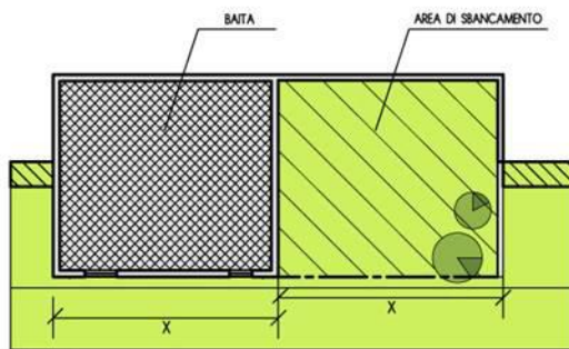
PIANTA
