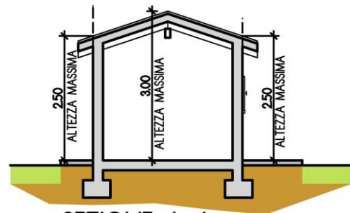
SEZIONE A-A
