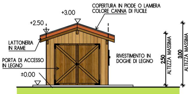
PROSPETTO FRONTALE
