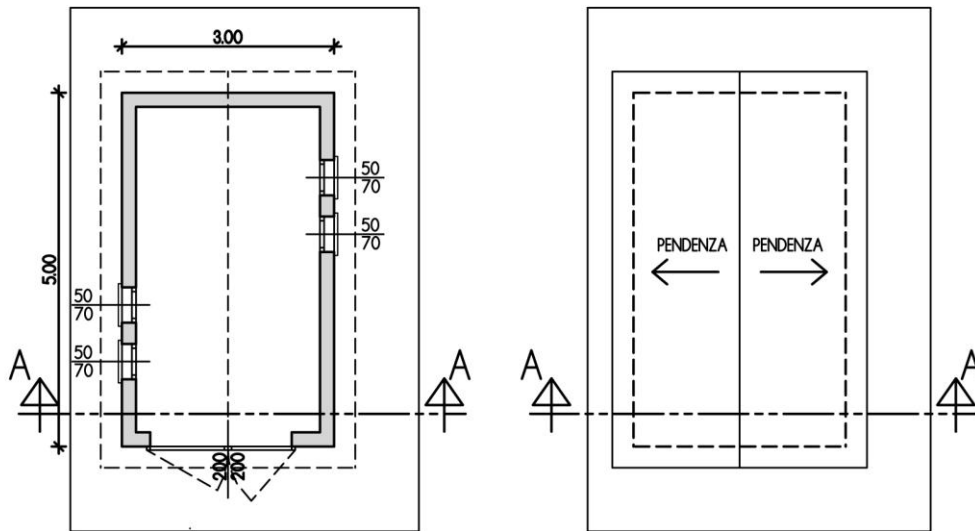
PIANTA STRUTTURA ACCESSORIA
