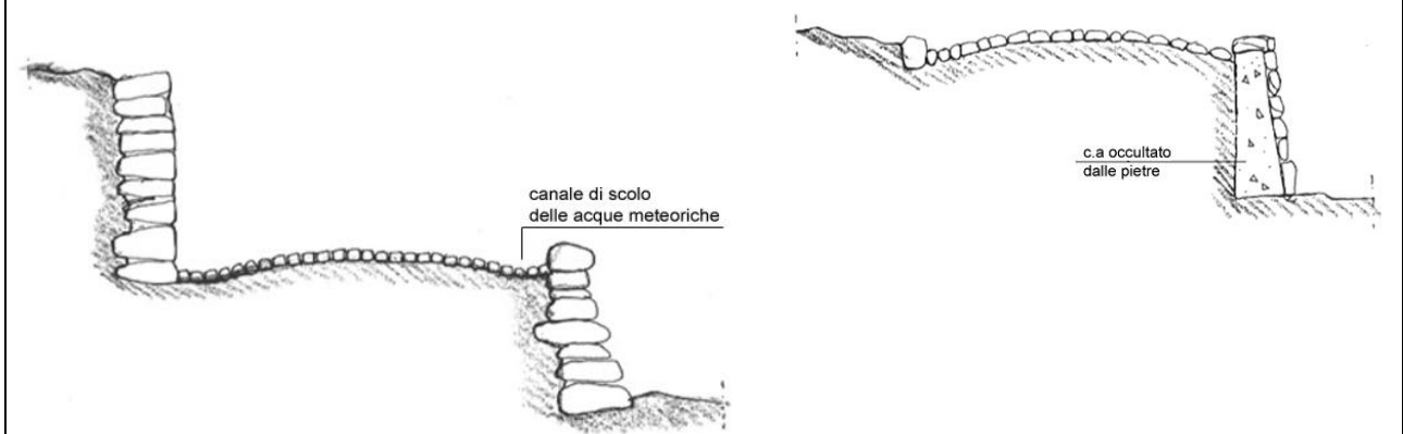
Nuove opere di finitura laterale
