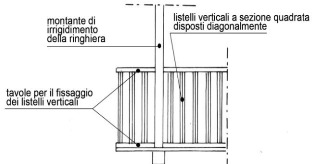
BALCONE INTERAMENTE IN LEGNO
