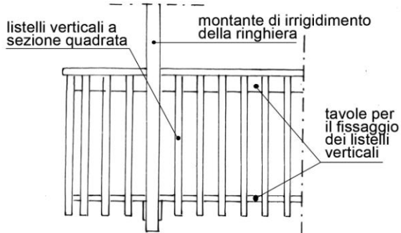
BALCONE INTERAMENTE IN LEGNO
