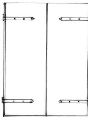
Scuri ad anta cieca
