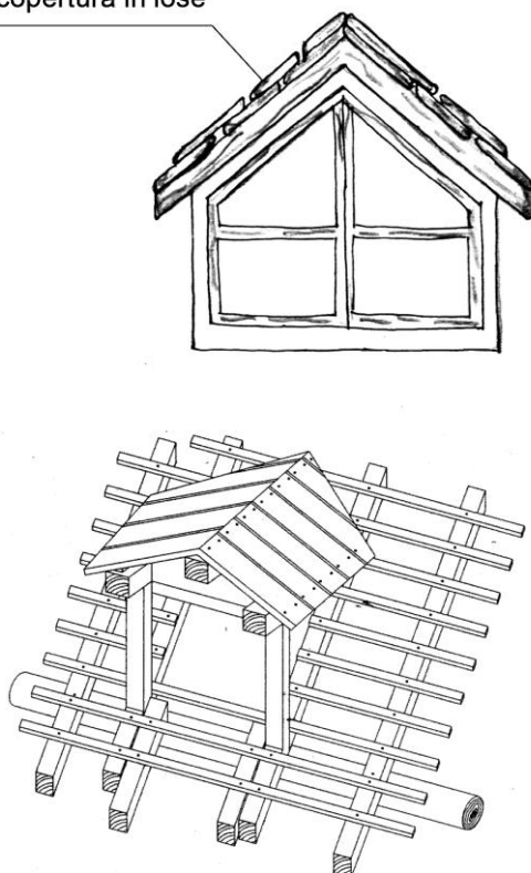
schema di abbaino a capanna
