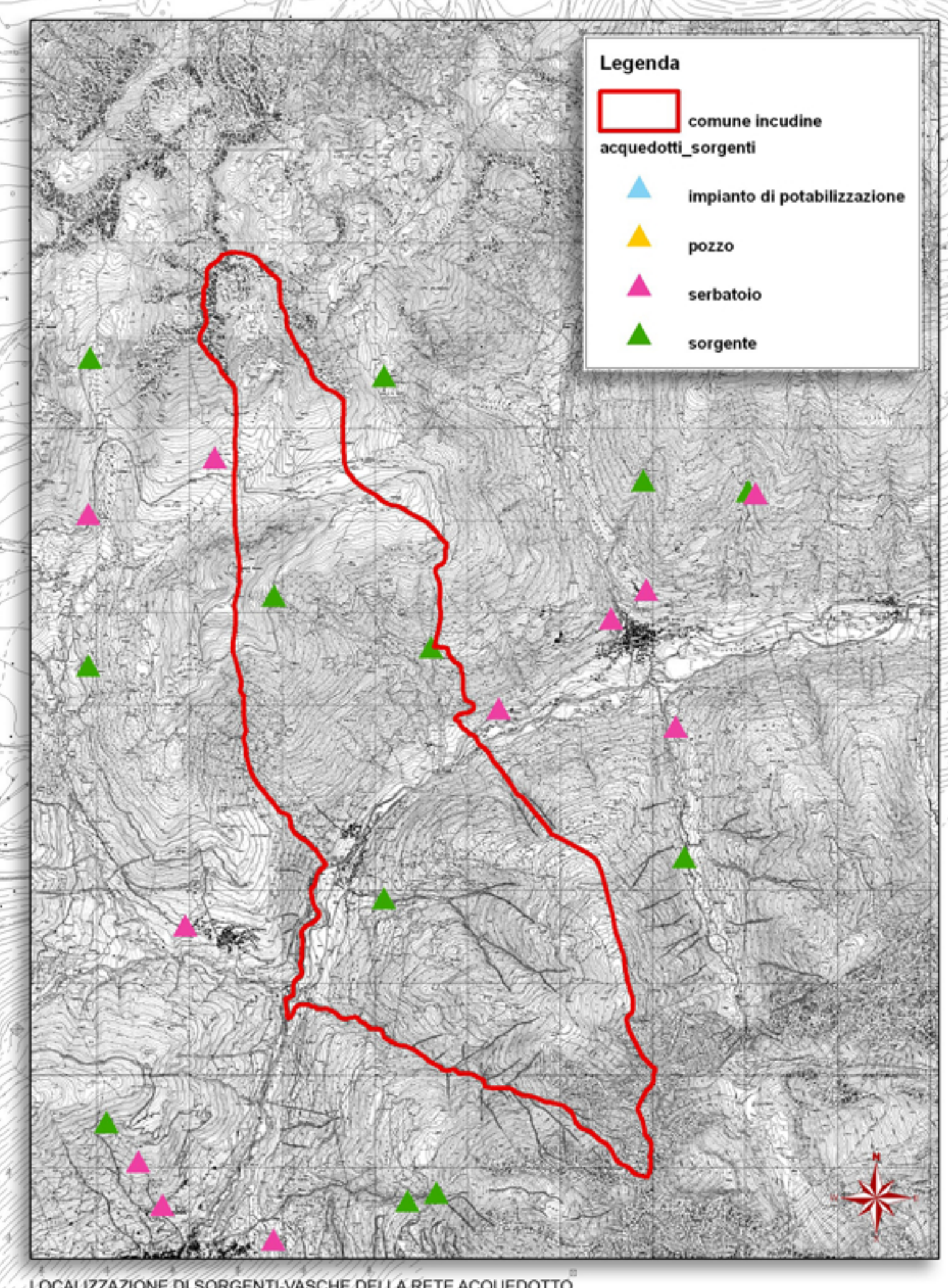
LOCALIZZAZIONE DI SORGENTI-VASCHE DELLA RETE ACQUEDOTTO SCALA 1:50.000
