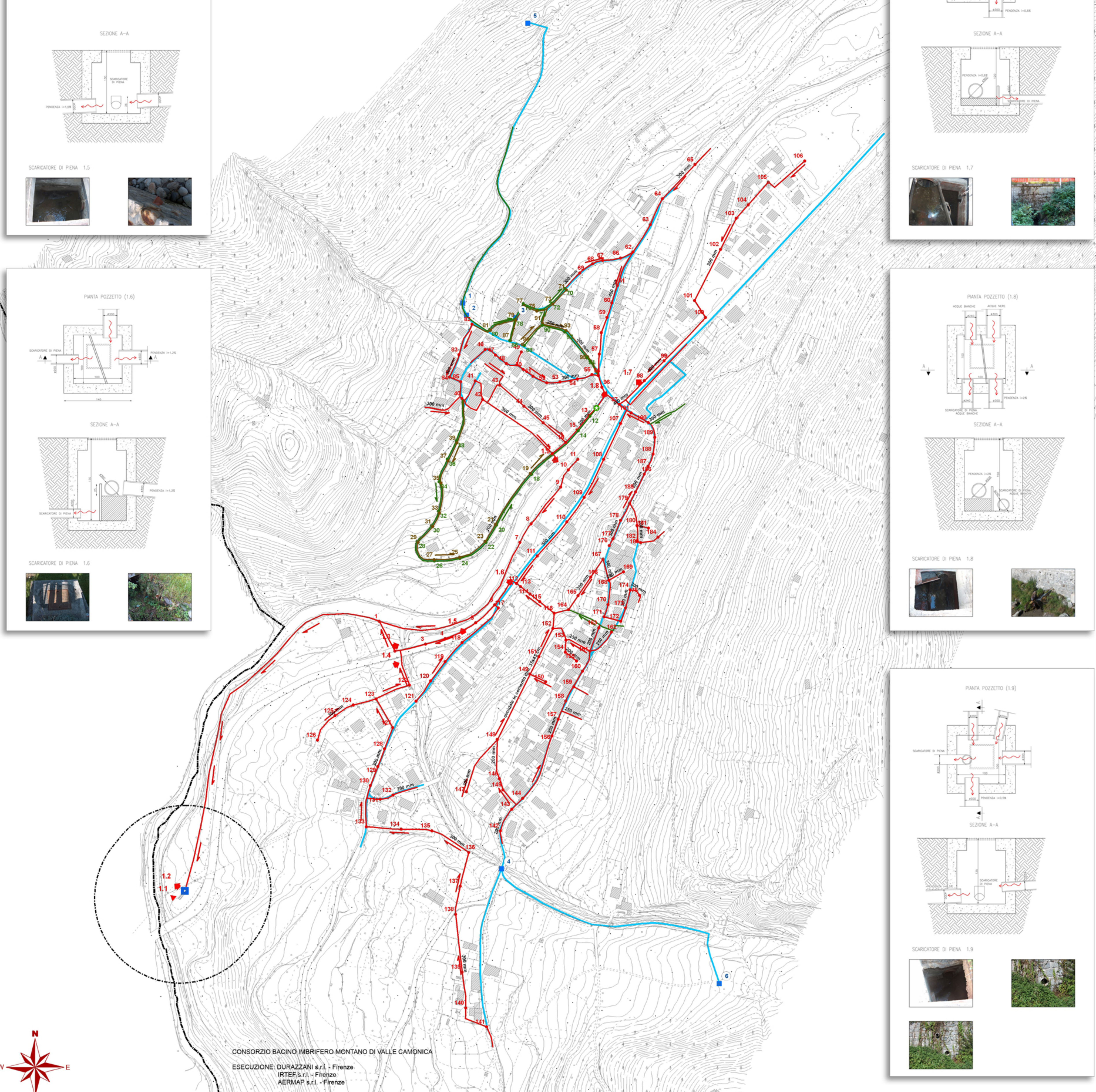
LOCALIZZAZIONE DI SORGENTI-VASCHE DELLA RETE ACQUEDOTTO SCALA 1:50.000
