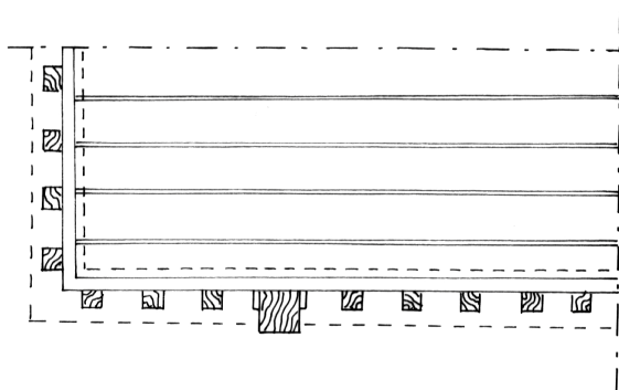
SEZIONE ORIZZONTALE - listelli verticali in legno a sezione quadrata
