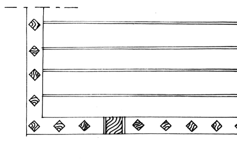
SEZIONE ORIZZONTALE - listelli a sezione quadrata disposti diagonalmente
