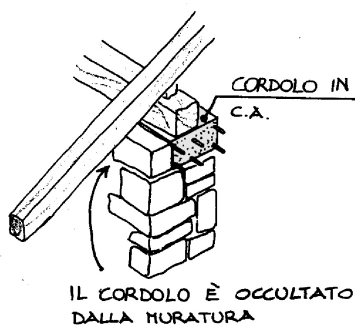
Particolare cordolo
