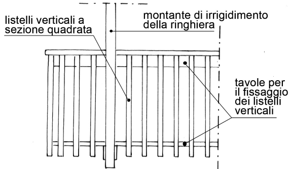
BALCONE INTERAMENTE IN LEGNO
